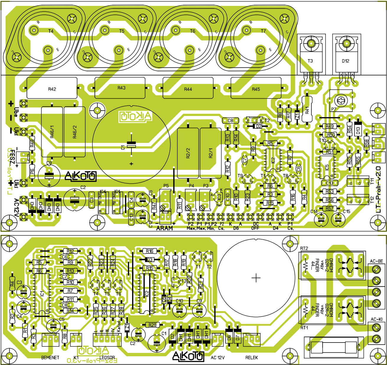
Labortap Profil007 kapcsolasa alapjan v2.0 VENTI RELE
