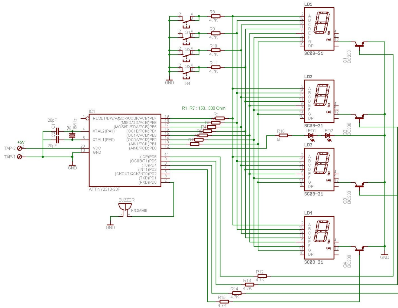
7 szegmenses LED kijelzős digitális óra. Attiny2313-as mikrokontrollerrel.
