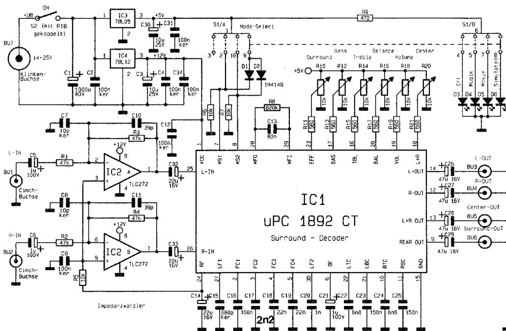
Bild 1: Schaltbild des ELV-Surround-Sound-Decoders SD 1000
