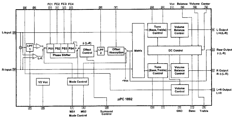
Bild 2: Interne Struktur des µPC1892CT
