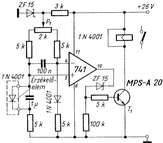
207. ábra. Differenciál-termométer (Motorola)
