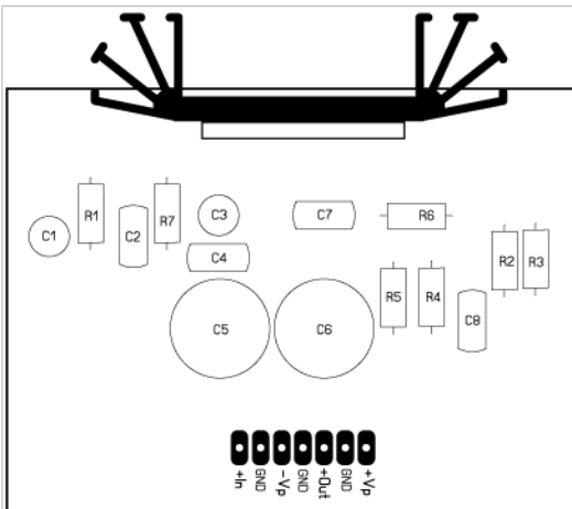
TOP-fólia
