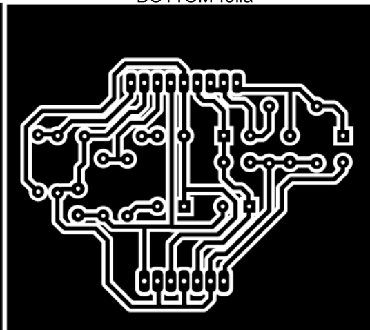
BOTTOM-fólia
