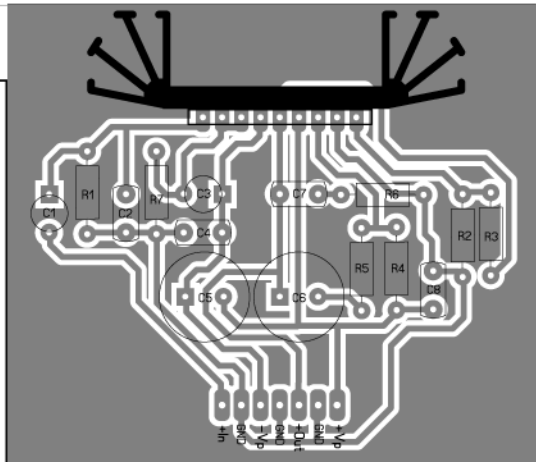
BOTTOM-fólia
