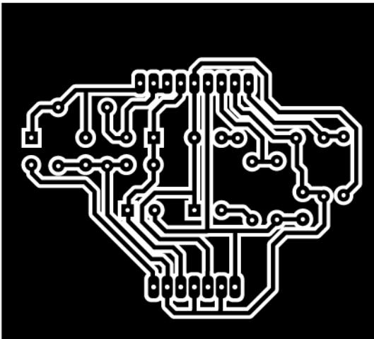
TOP-fólia
