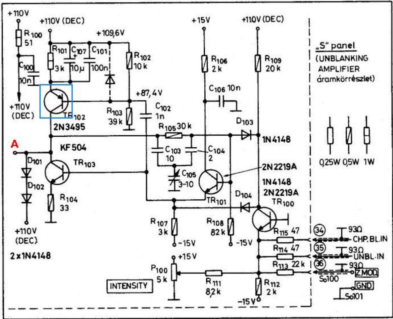
3. ábra. A kivilágosító erősítő kapcsolási rajza
