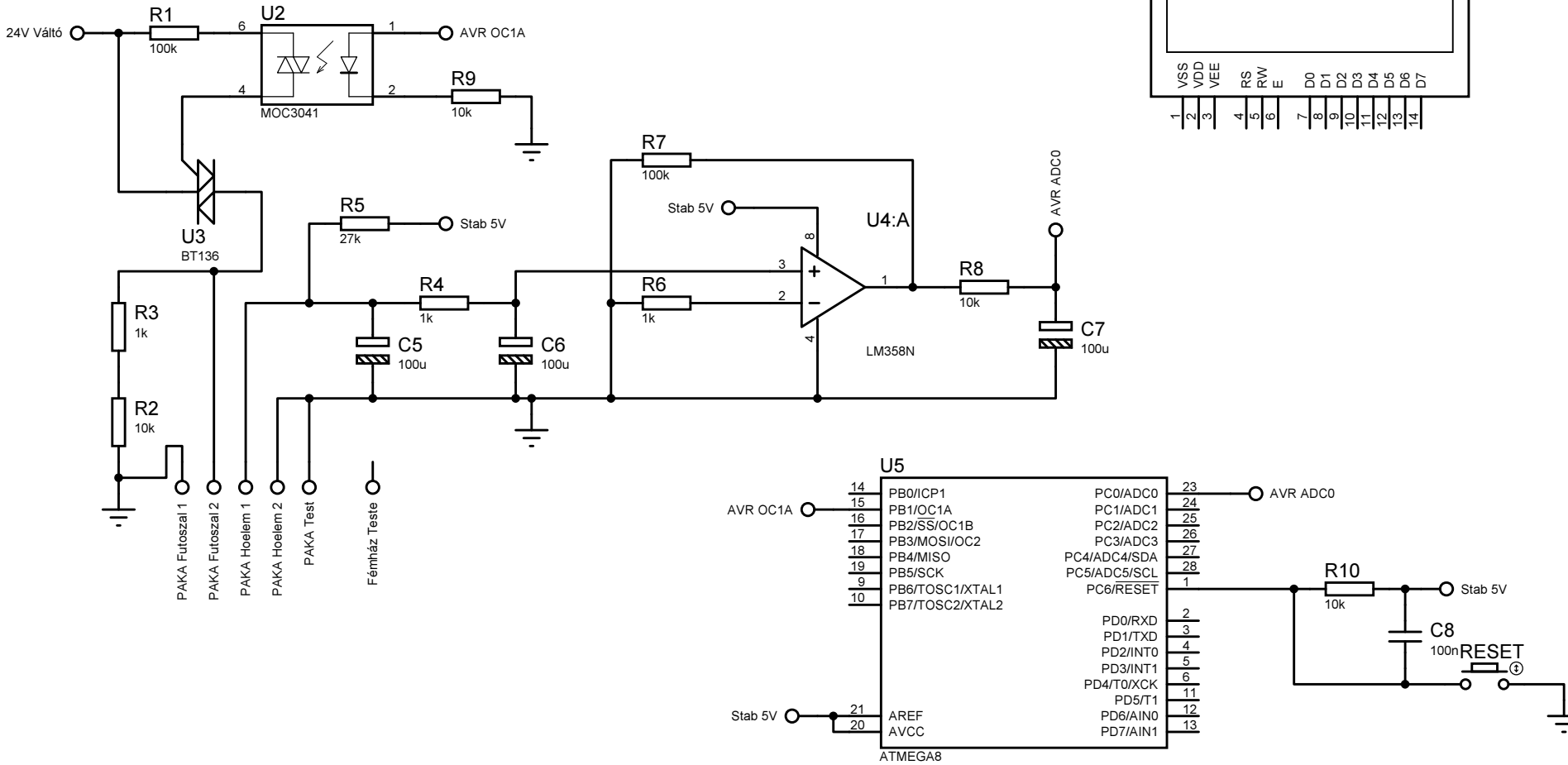
LCD1 LM016L
