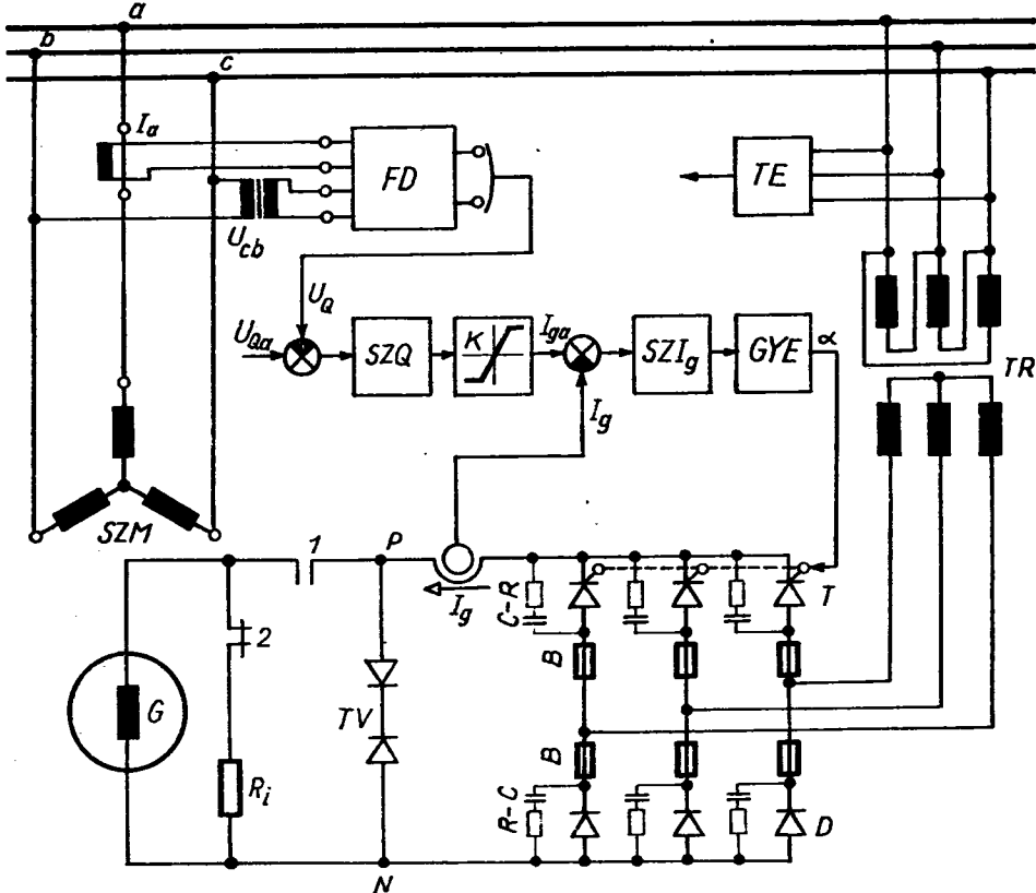
8.21. ábra. Szinkronmotor állandó meddő teljesítményre való szabályozása
