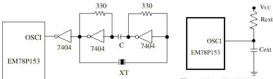
图 16: 外部RC振荡器模式电路
