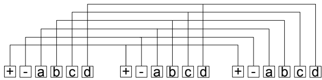
Aljzat kiosztás
