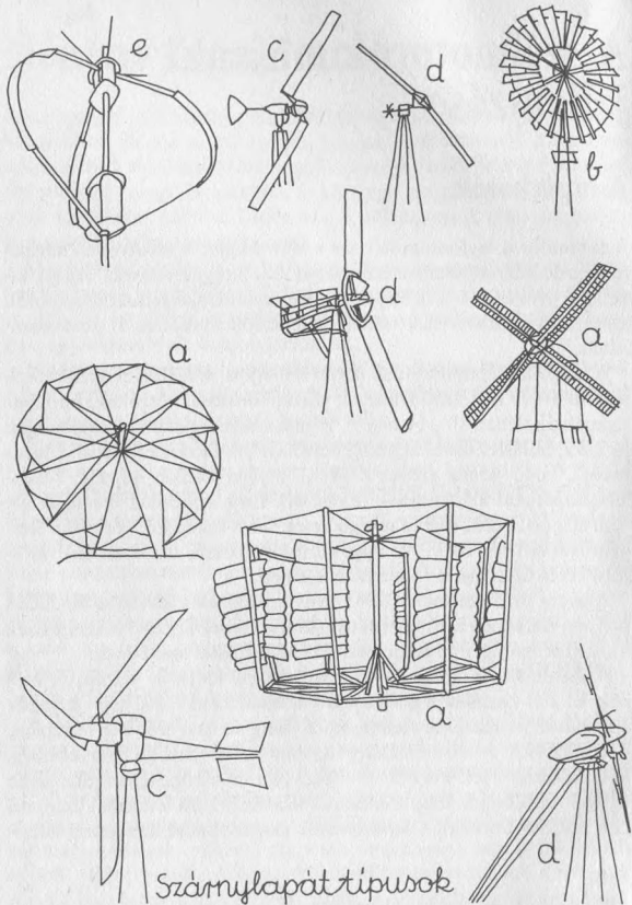
1. ábra: Különböző szélmotorok: a) vitorla lapátozású típusok; b) sűrű lapátozású, amerikai típus; c) két- és háromlapátos, gyors járású típusok; d) két- és háromlapátos szélmotorok; e) függőleges tengelyű „darrieus” típusok
