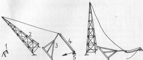
7. ábra. Szélmotor állványzatának felállítása segédállvánnyal: 1 — tartók; 2 — állvány 3 — segédállvány; 4 — csörlő; 5 — cölöp
