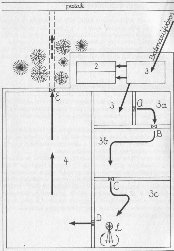
5. ábra. Szennyvíztelep elrendezési vázlata: 1 — ülepítő; 2 — szikkasztó; 3, 3a, 3b és 3c — előtároló medencék; A, B, C, D és E — zsilipek; L — levegőztetőkereket hajtó szélmotor; 4 — utótároló
