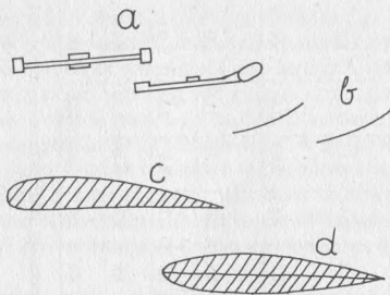
2. ábra. Jellemző lapáttípusok: a) régebbi (szélmalom); b) hagyományos sűrű lapátos; c) és d) újabb, gyors járású, propelleres típusok (konvex és bikonvex profilok)
