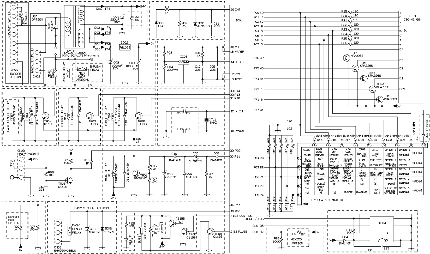
N2LED1 SCHEMATIC
