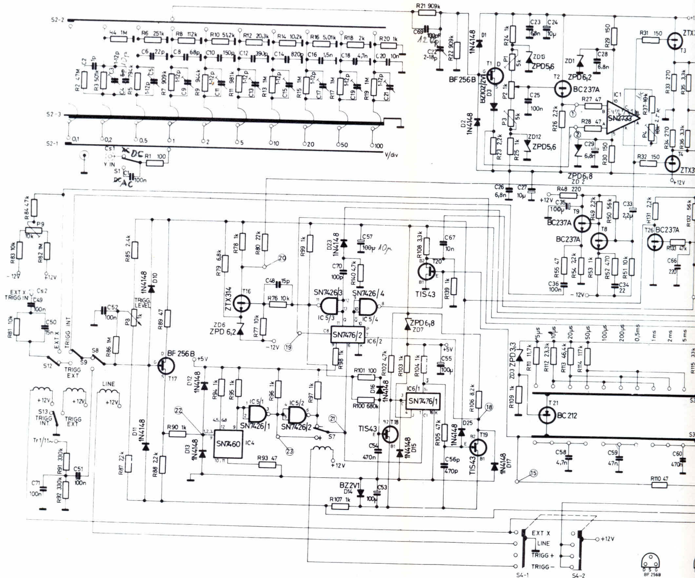
2. melléklet Elvi kapcsolási rajz
