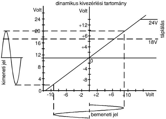
3-as ábra: ICP ® érzékelők kivezérelhetősége a táplálás függvényében
