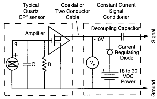
2-es ábra: tipikus mérőkör-összeállítás ICP ® érzékelő esetén
