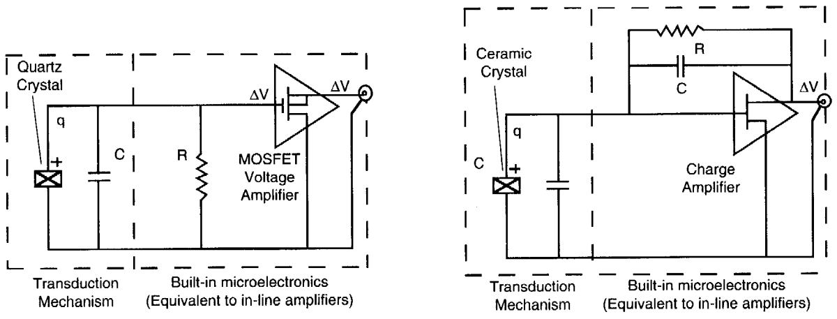
kvarc-alapú piezoelektromos érzékelő belső felépítése kerámia-alapú piezoelektromos érzékelő belső felépítése
