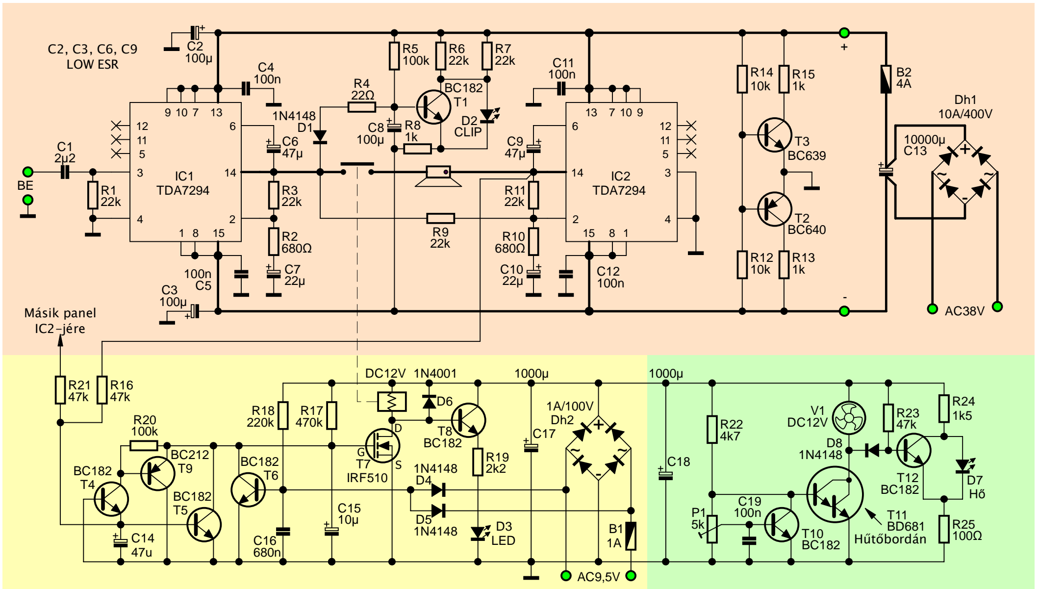
"Egytápos" híd, Reloop elképzelése alapján, CLIP jelzéssel, védelemmel és hőfokfüggő ventilátor vezérléssel AKOTÓ-s ábrarajolat (v1.1).
