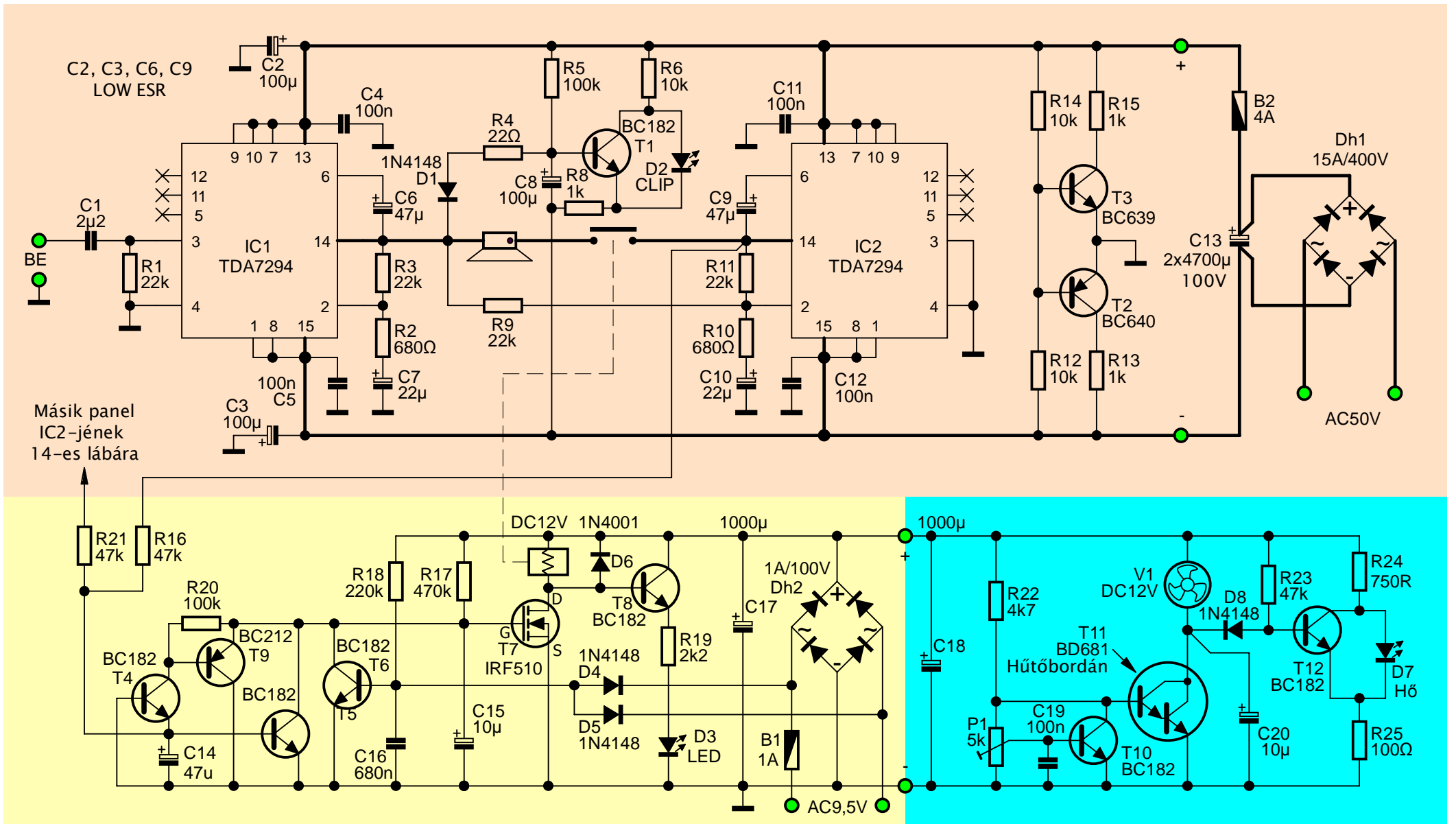
"Egytápos" híd, Reloop elképzelése alapján, CLIP jelzéssel, védelemmel és hőfokfüggő ventilátor vezérléssel AKOTÓ-s ábrázolat (v1.1b).
