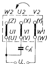
4.41. ábra. Csillagkapcsolású motor üzemeltetése egyfázisú hálózatról
