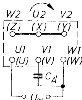
4.41. ábra. Csillagkapcsolású motor üzemeltetése egyfázisú hálózatról
