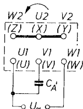
4.41. ábra. Csillagkapcsolású motor üzemeltetése egyfázisú hálózatról
