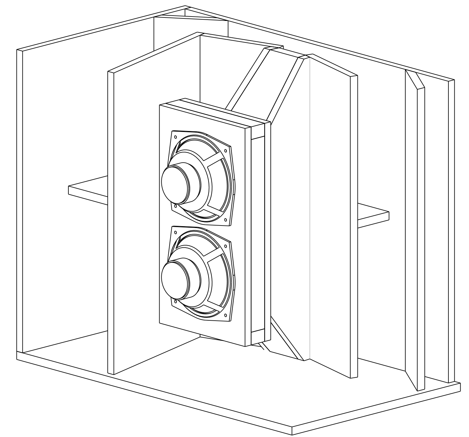
Térbeli nézet levett oldal , előlap,belső tereiőlappal
