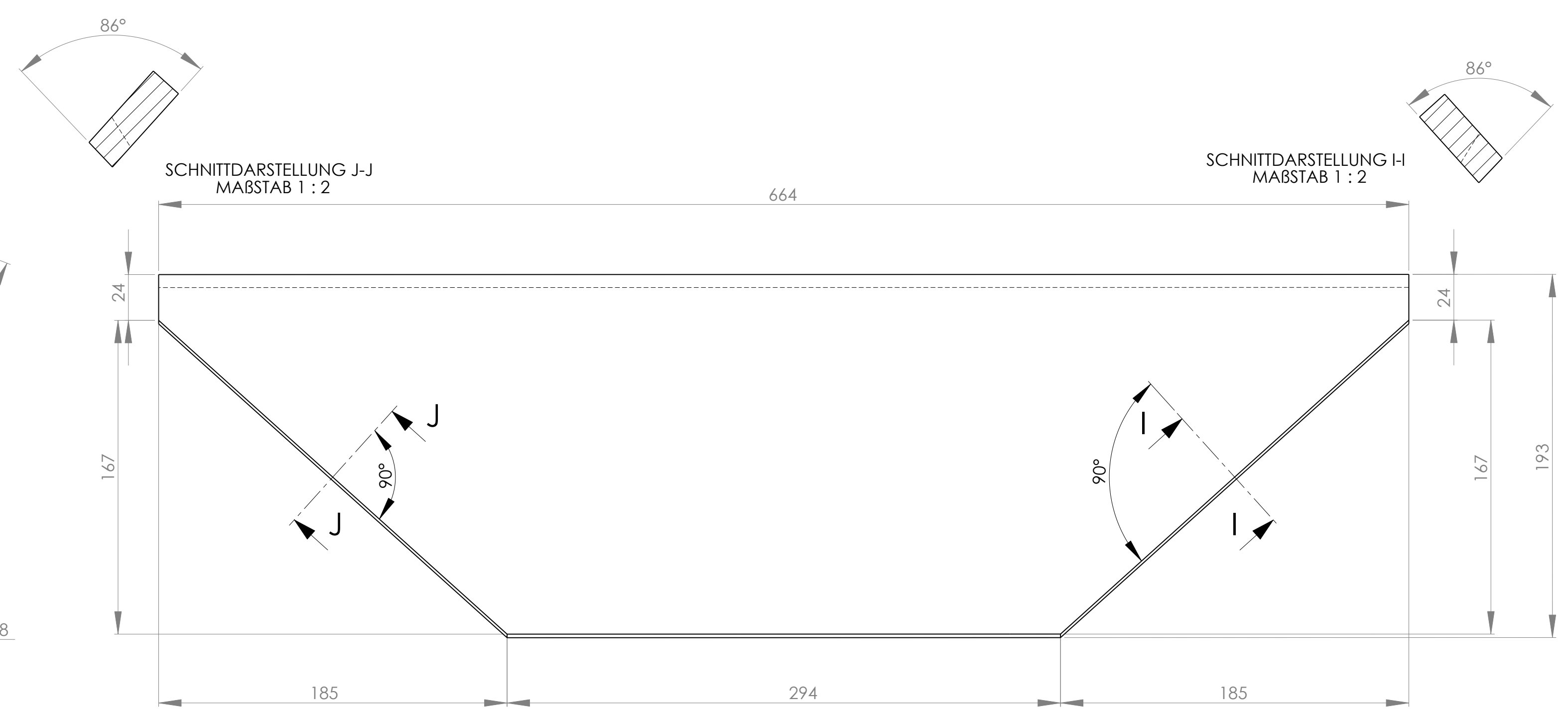
ANSICHT H MAßSTAB 1 : 2
