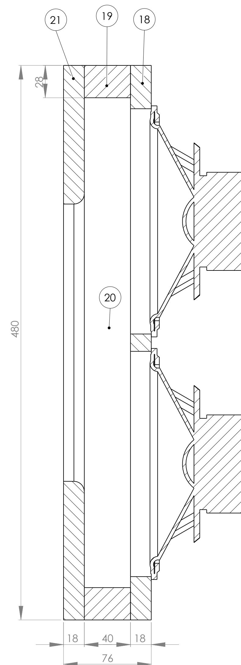
SCHNITTDARSTELLUNG E-E MABSTAB 1 : 2
