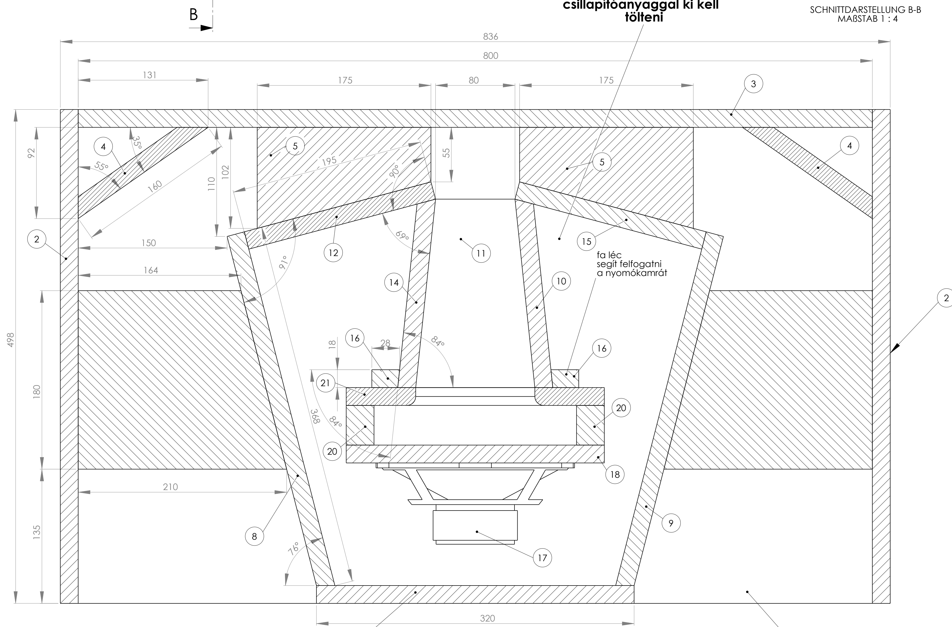
SCHNITTDARSTELLUNG A-A MÁBSTAB 1 : 2
