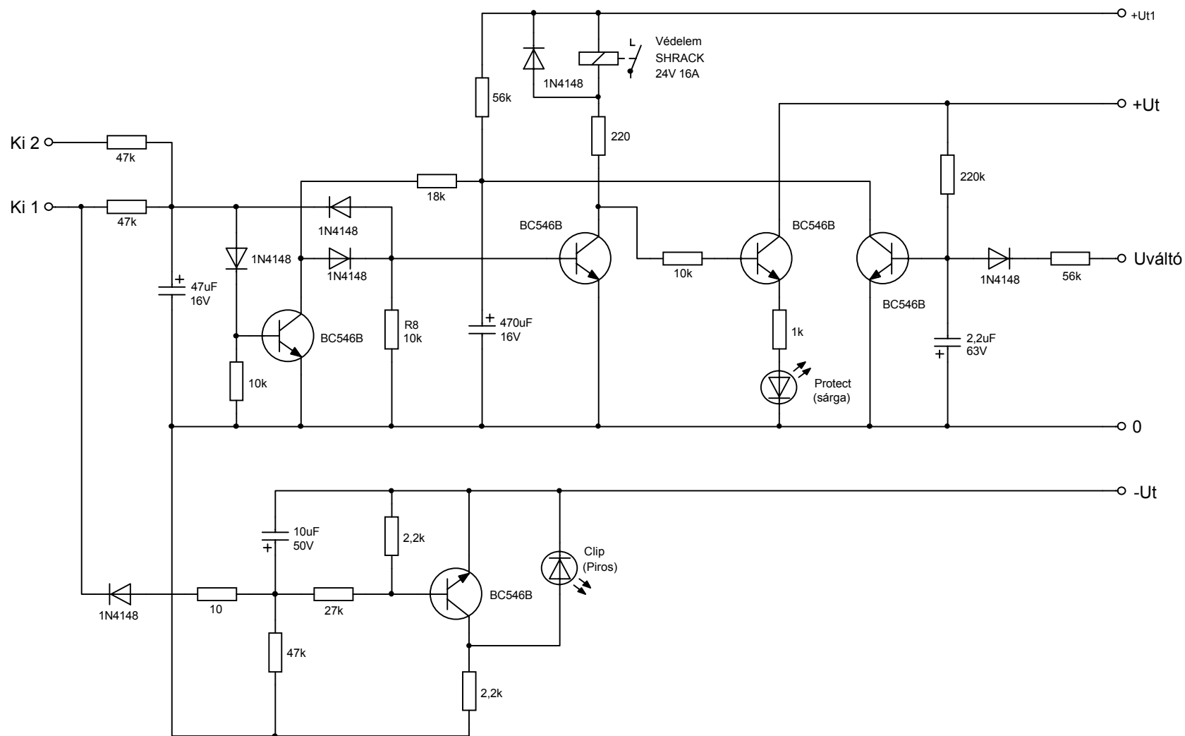
REFLEX RX-500 Végerősítő - Védelmi és csúcsértékjelző áramkör (egyik csatorna)
