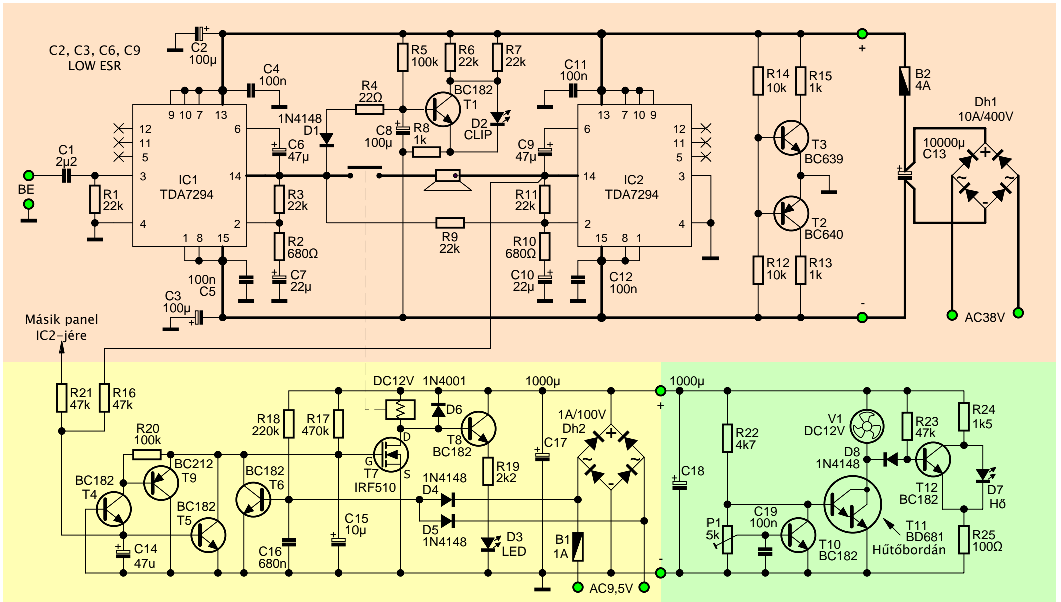
"Egytápos" híd, Reloop elképzelése alapján, CLIP jelzéssel, védelemmel és hőfokfüggő ventilátor vezérléssel AKOTÓ -s ábrázolat (v1.1).
