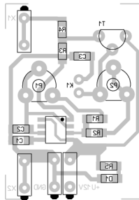
Beültetés.oldal
