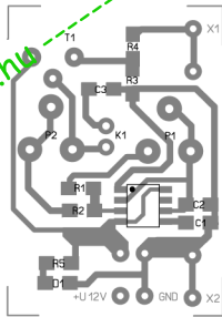
Fólia.SMD.oldal
