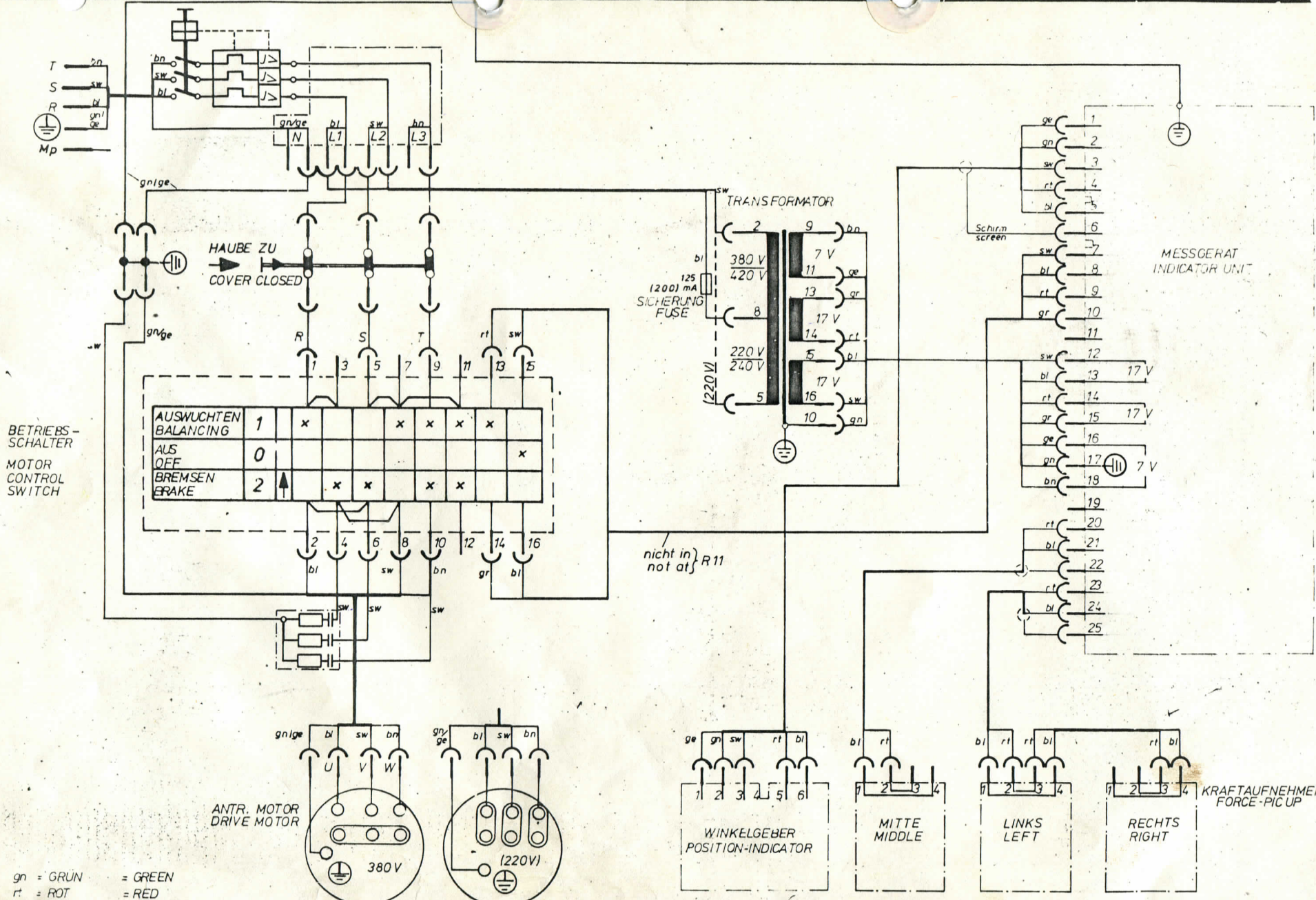
SCHALTPLAN, RADAUSWUCHTMASCHINE CIRCUIT DIAGRAM, WHEEL - BALANCER (220)380 V 50Hz 3PH AC BRAKE Sonderausführung
