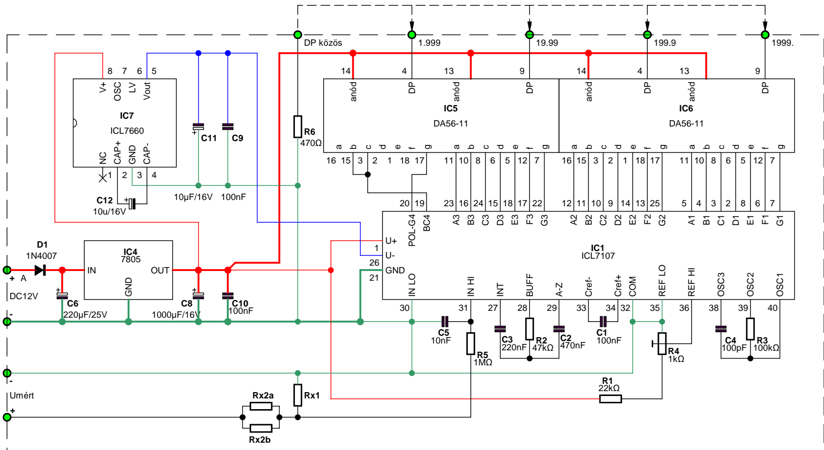
3,5 digites, 200mV-os (199,9) kijelző, bementi osztóval DC12V-ről, gépkocsiban való méréshez. Alkotó-s elképzelés
