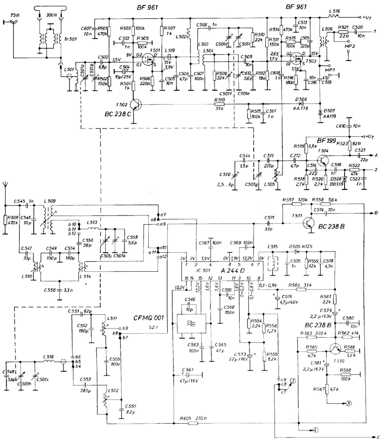
92. ábra Az ST 1025 típusú rádiótuner áramköreinek kapcsolási vázlata
