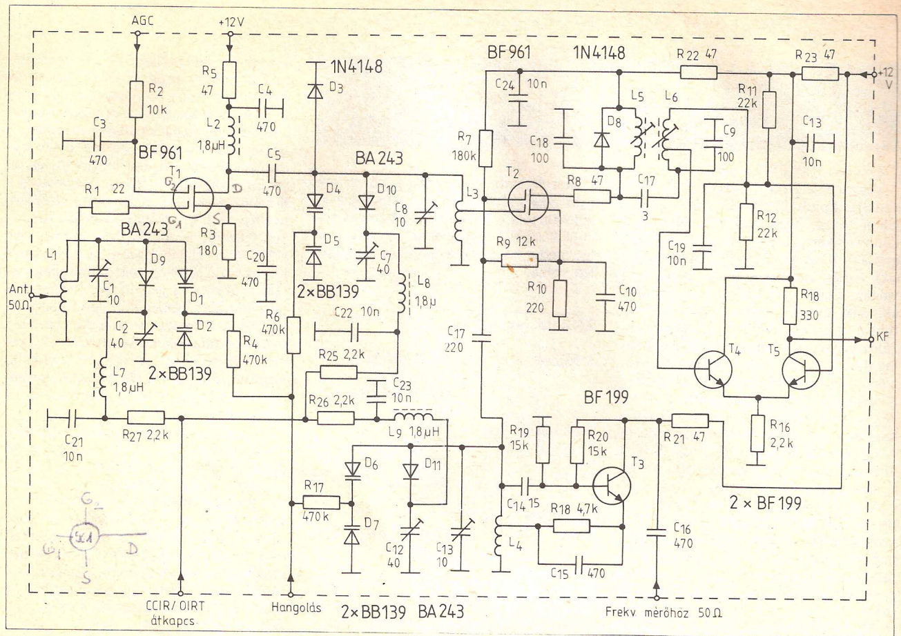
2. ábra. Az RF-egység kapcsolási rajza
