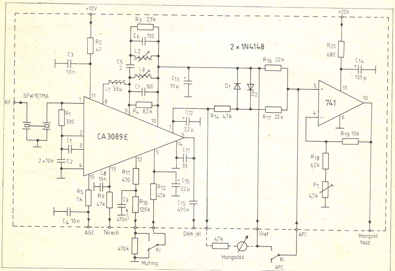
3. ábra. A KF-egység kapcsolási rajza
