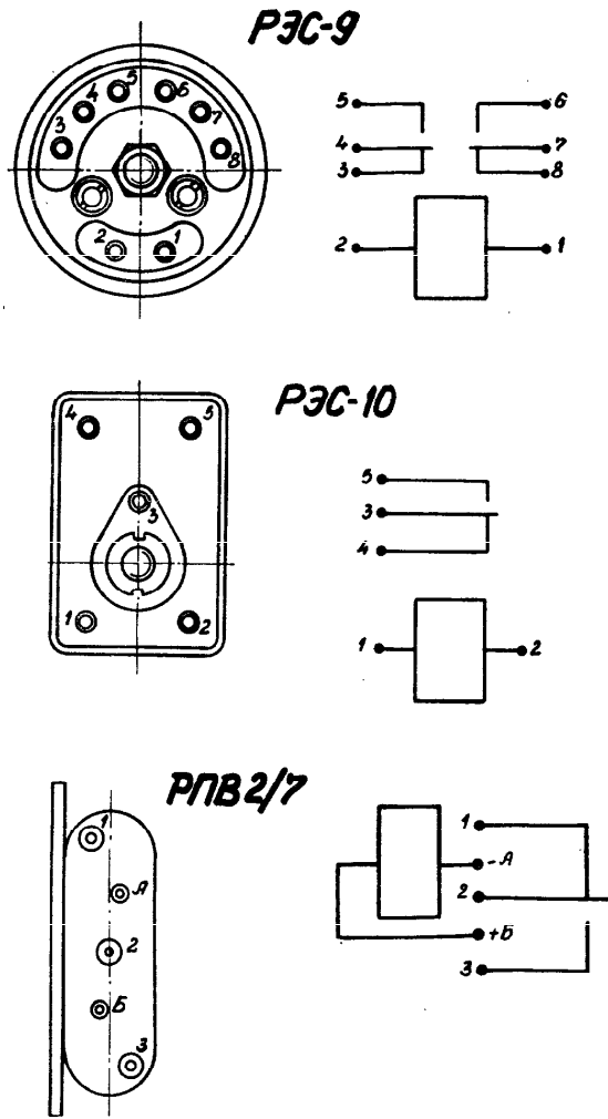
Приложение 8. Цоколевка реле РЭС-9, РЭС-10 и РПВ2/7
