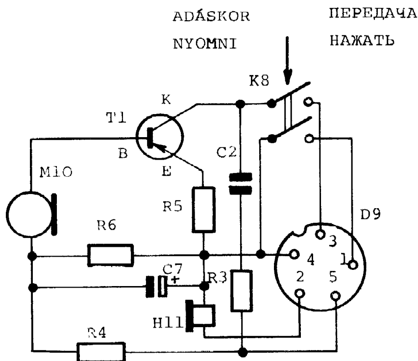
МИКРОТЕЛЕФОННАЯ ГАРНИТУРА. Схема принципиальная электрическая MIKROTELEFON KÉSZLET. Elektromos elvi kapcsolási rajz
