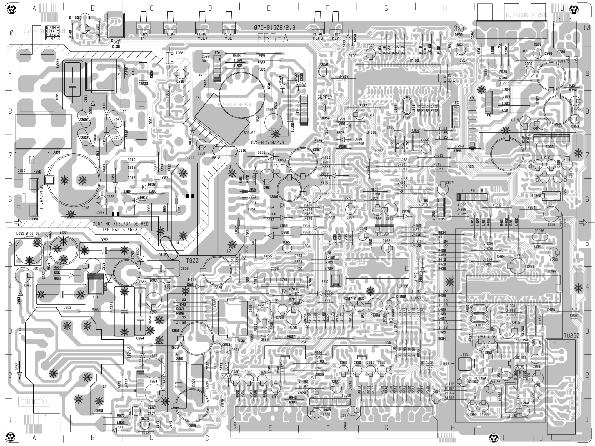
P.C.B. CIRCUITO GENERAL CARA COMPONENTES MAIN P.C.B. COMPONENTS SIDE P.C.B. PANNELLO PRINCIPALE LATO COMPONENTI
