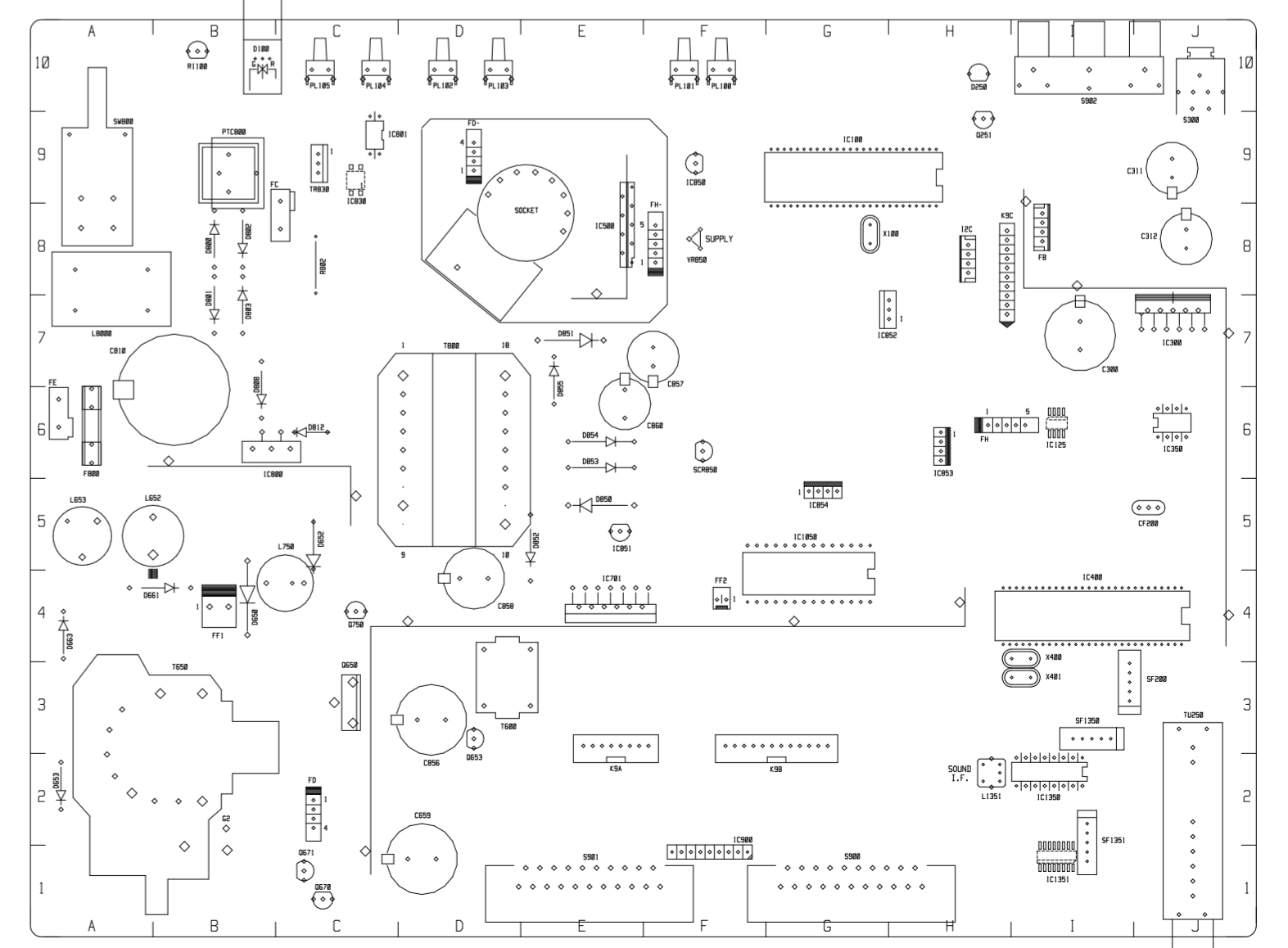
LOCALIZACION DE COMPONENTES CIRCUITO GENERAL MAIN CIRCUIT COMPONENTS LOCATION LOCALIZZAZIONE DI COMPONENTI PANNELLO PRINCIPALE
