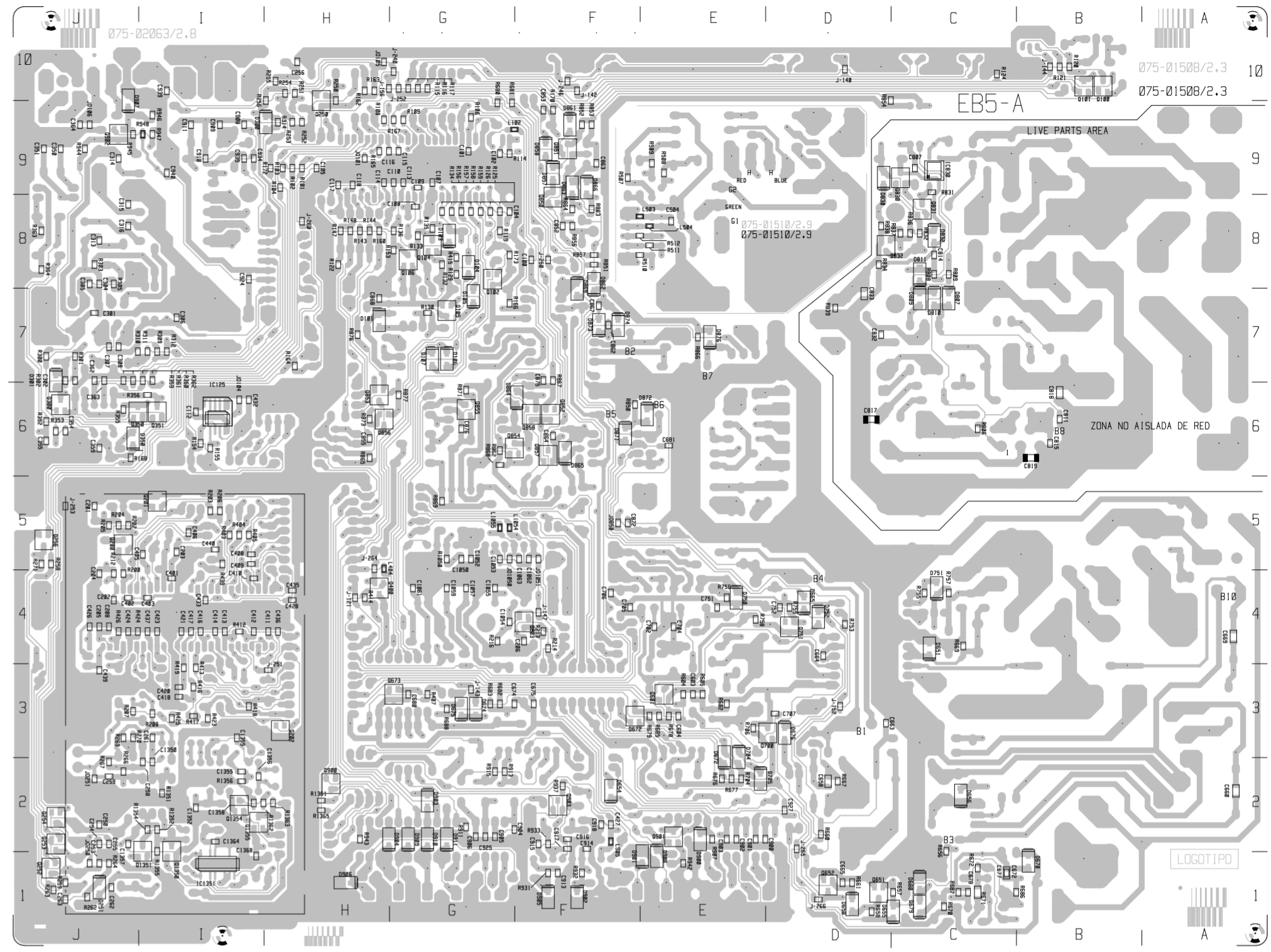
P.C.B. CIRCUITO GENERAL CARA SOLDADURAS MAIN P.C.B. SOLDER SIDE P.C.B. PANNELLO PRINCIPALE LATO SOLDATURE
