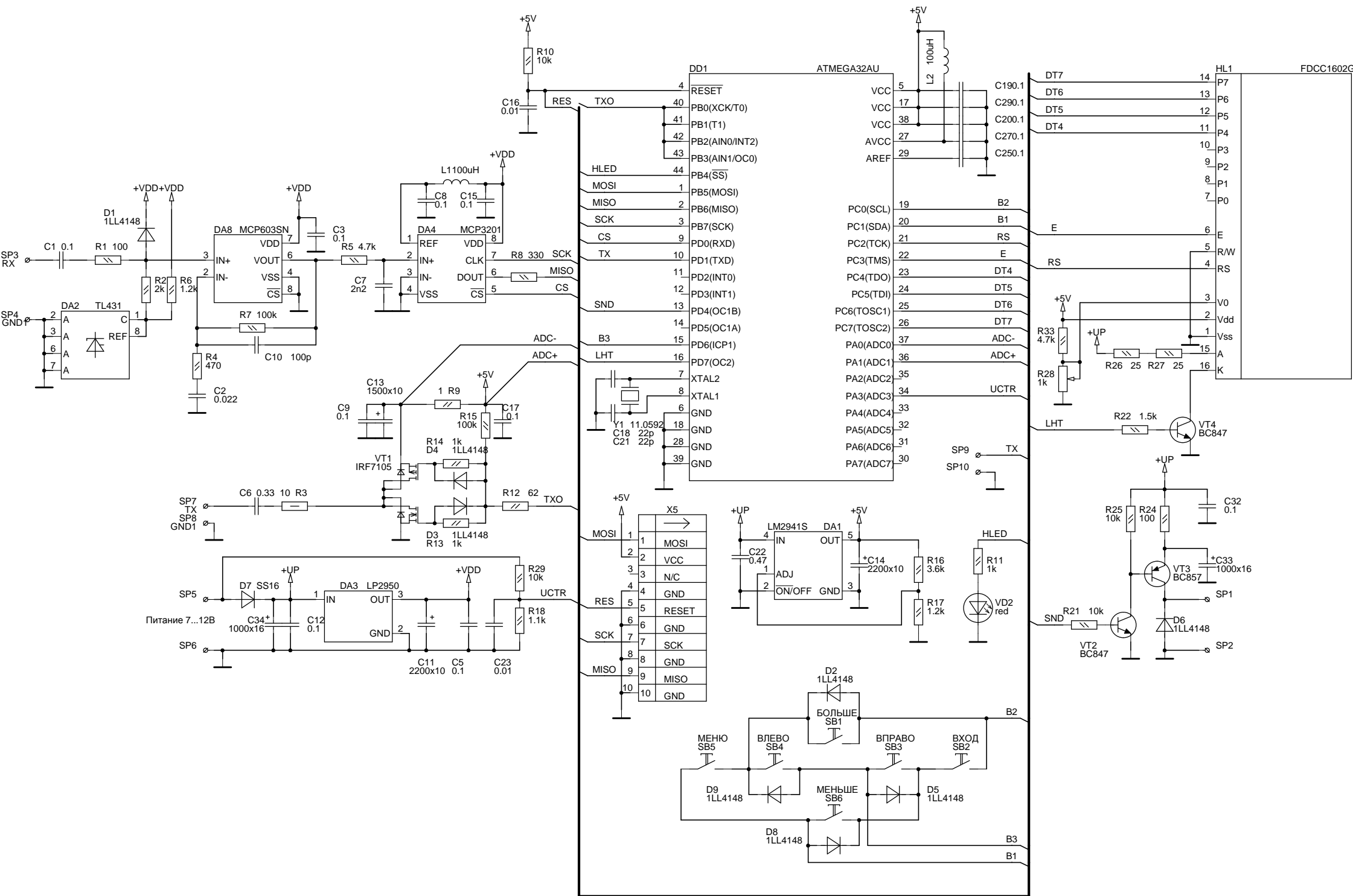
Схема ИВ-металлоискателя "Quasar". Автор проекта Andy_F. Рисовал verybed. 10/05/2012
