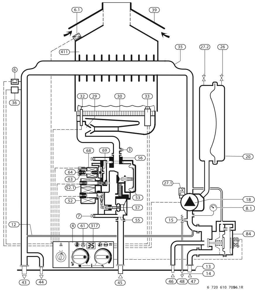
11. ábra Kéményes fűtőkészülék beépített előnykapcsolással (Nr. 905) indirekt tároló fűtéséhez
