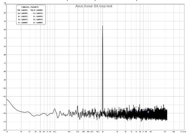
DS 44kHz THD=0,0032%, THD+N=0,0299%
