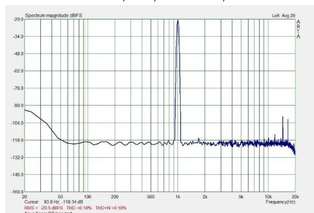
DS 192kHz THD=0,18%, THD+N=0,18%
