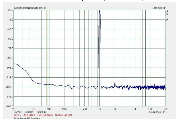
AISO 192kHz THD=0,026%, THD+N=0,12%
