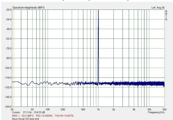
DS 44kHz THD=0,0029%, THD+N=0,027%
