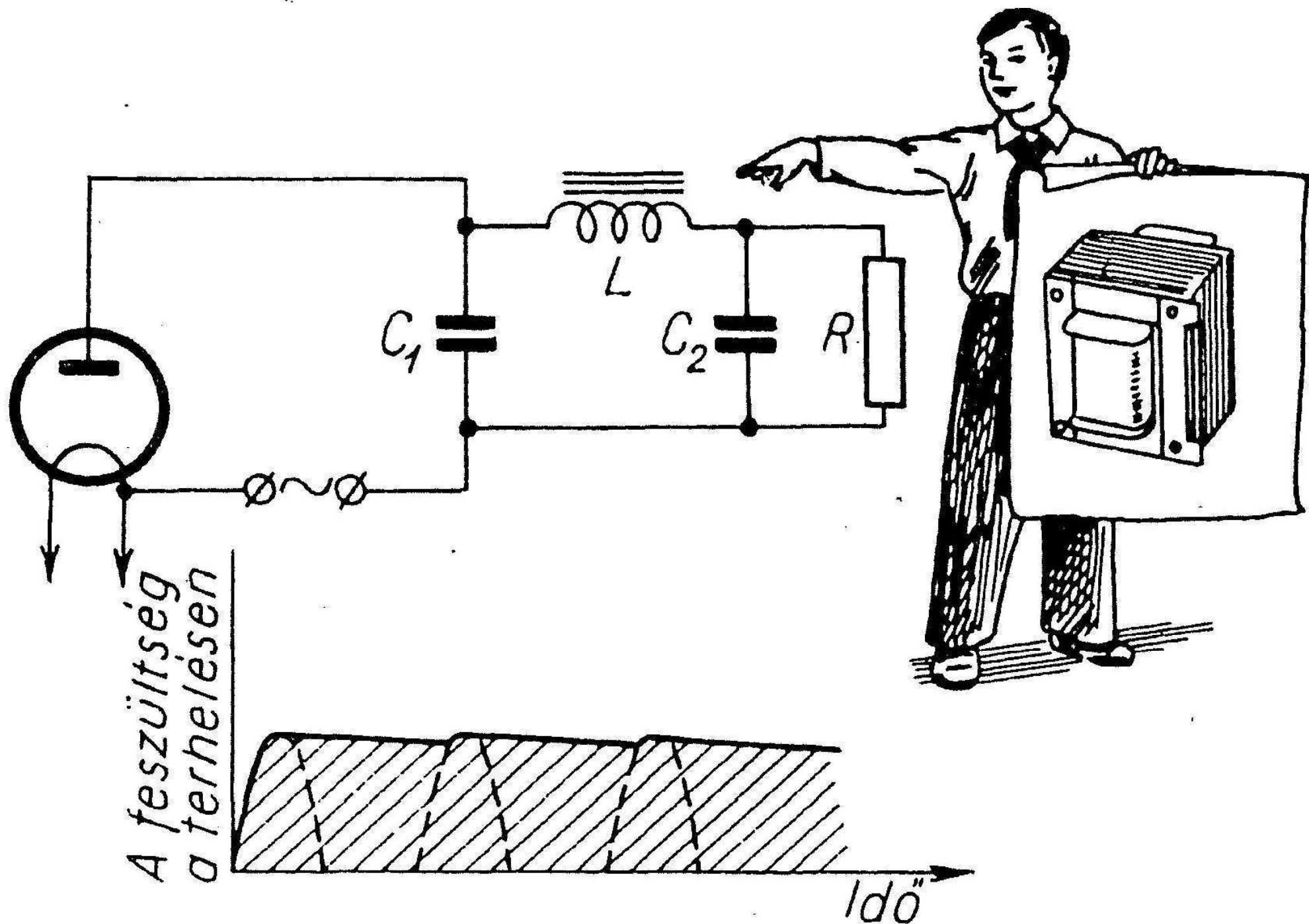
28. ábra. Lüktető egyenáram simítása LC szűrővel
