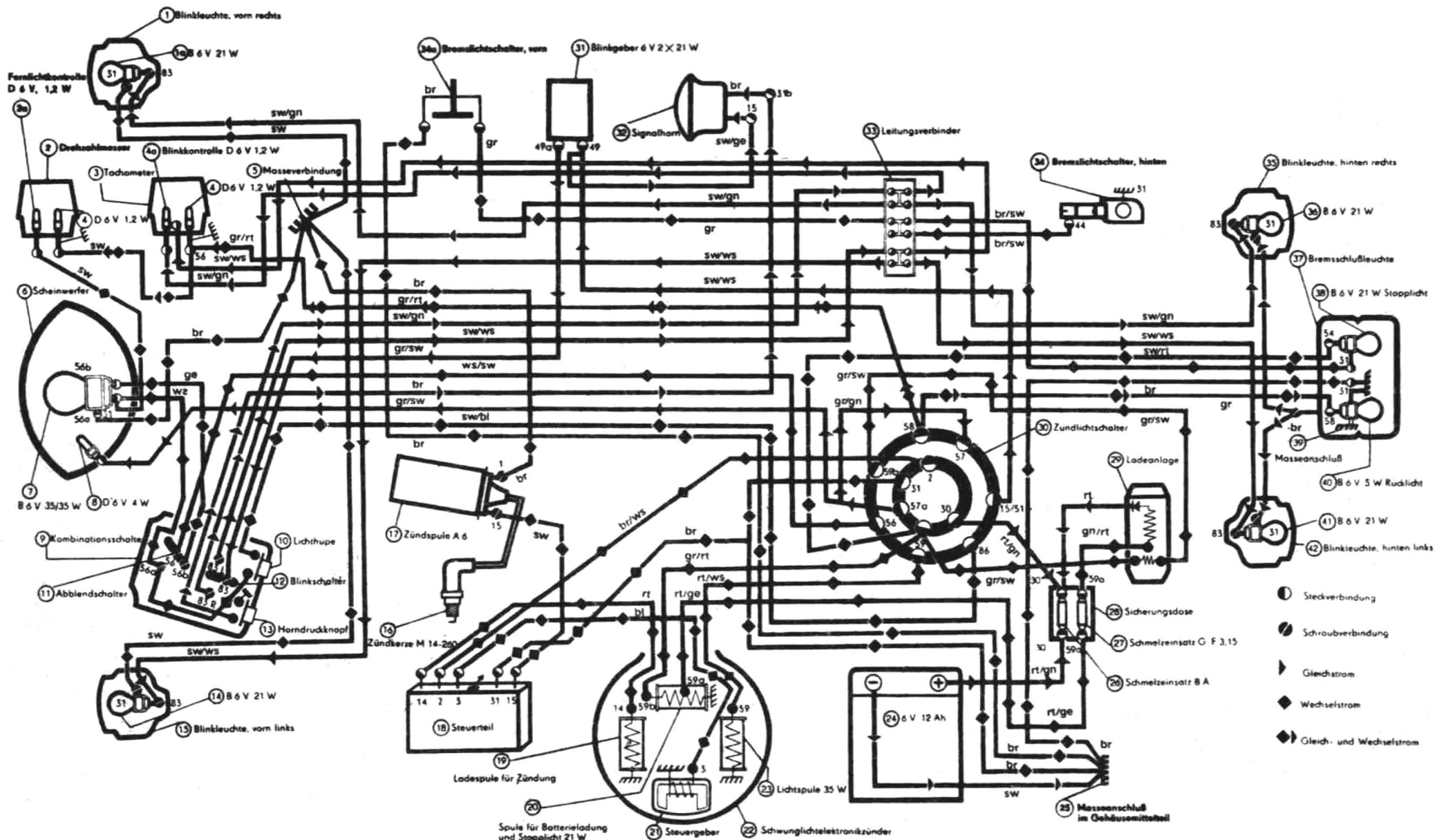
Schaltplan S51 B2-4, S51 E und S51 C
