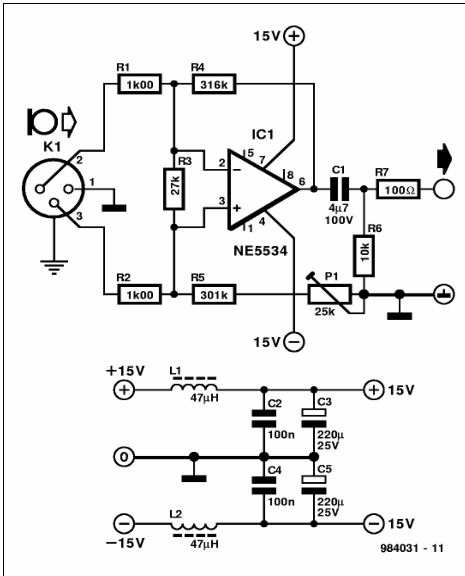
Simetrikus Mikrofonerősítő
