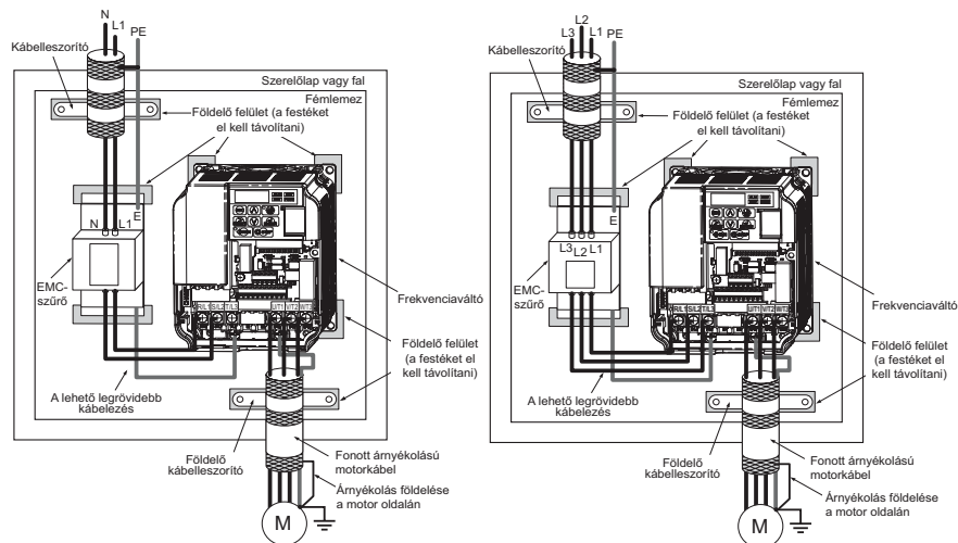
Az egy- és a háromfázisú egységek bekötése az EMC-szabványoknak megfelelően
