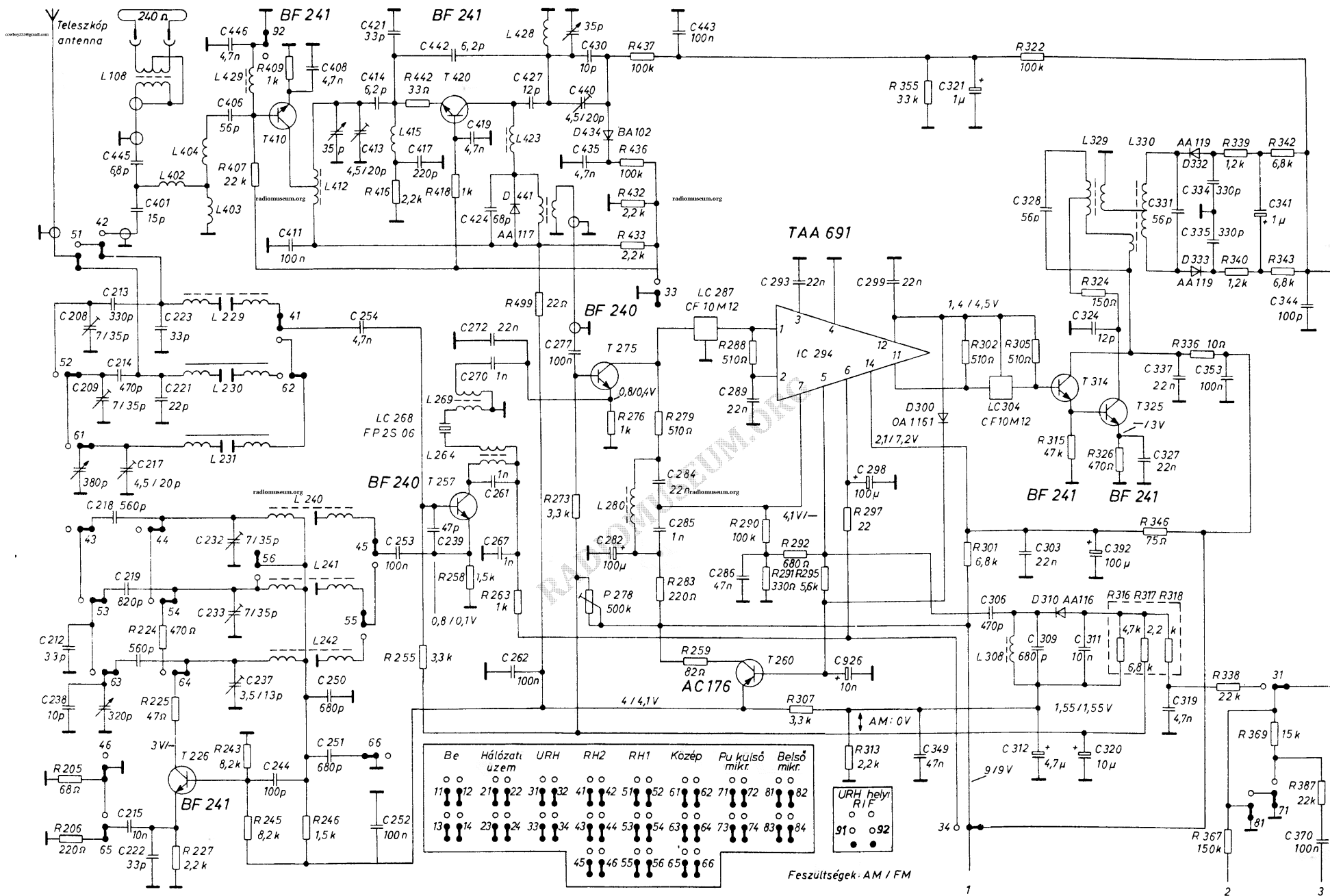
Az RM-4624 rádióész áramköreinek kapcsolási vázlatja
