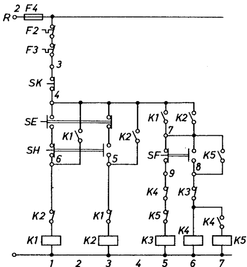
4.10. ábra. Pólusátkapcsolós hajtás kétféle fordulatszámra, két forgásirányra
