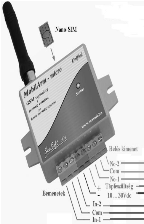
GSM átjelző 1.zóna – impulzusos kulcsos kapcsoló (5.zóna nem használt)
