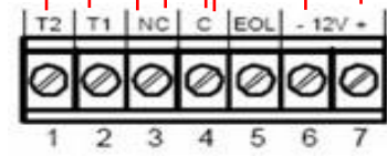
DSC LC-100 infra nappali 2.zóna – 2. késleltetett (6.zóna nem használt)
