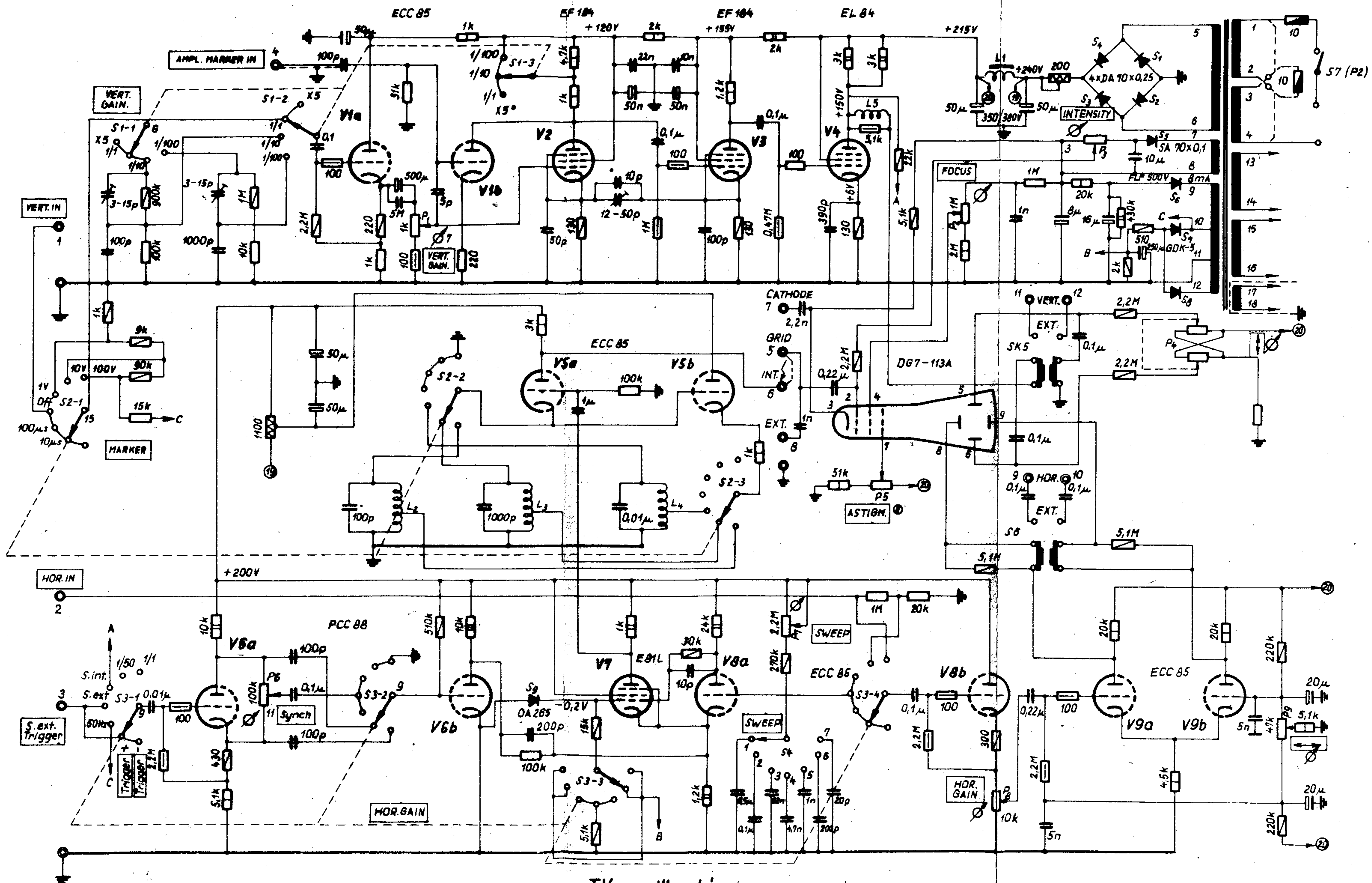
TV. oszcilloszkóp. (HIR.KTSZ TR 4302)
