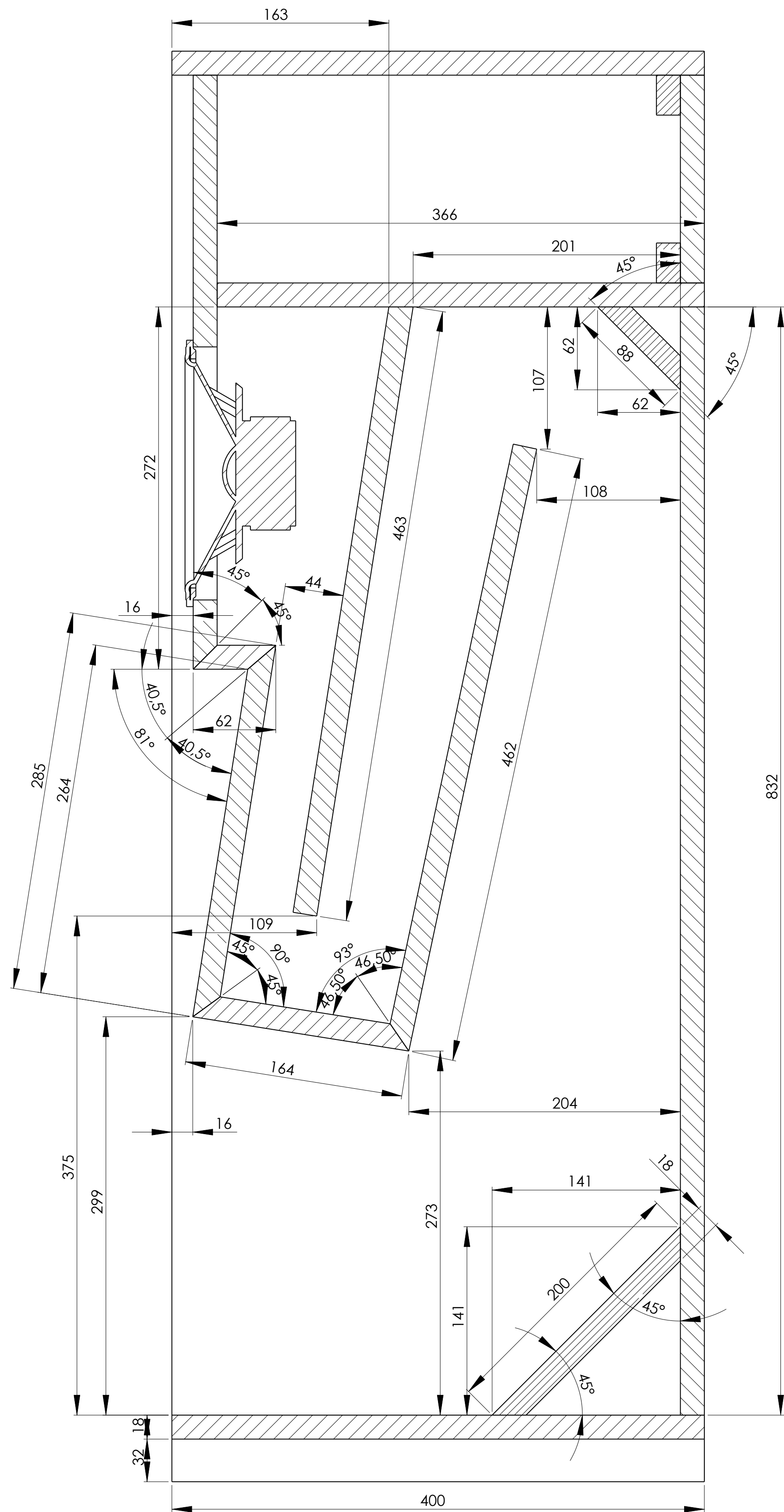
SCHNITTDARSTELLUNG A-A MÄßSTAB 2 : 5
