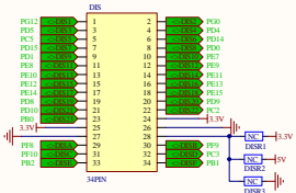
显示接口
