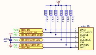
mSD卡
