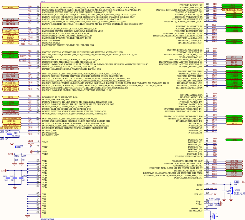
MCU
