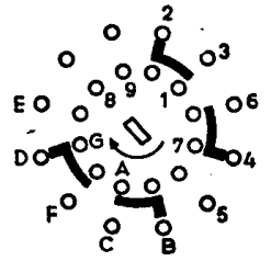
Ingelen Columbus 53 (ZF: 451 kHz bzw. 459 kHz)
