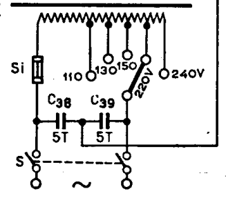
Ingelen Columbus 53 (ZF: 451 kHz bzw. 459 kHz)
