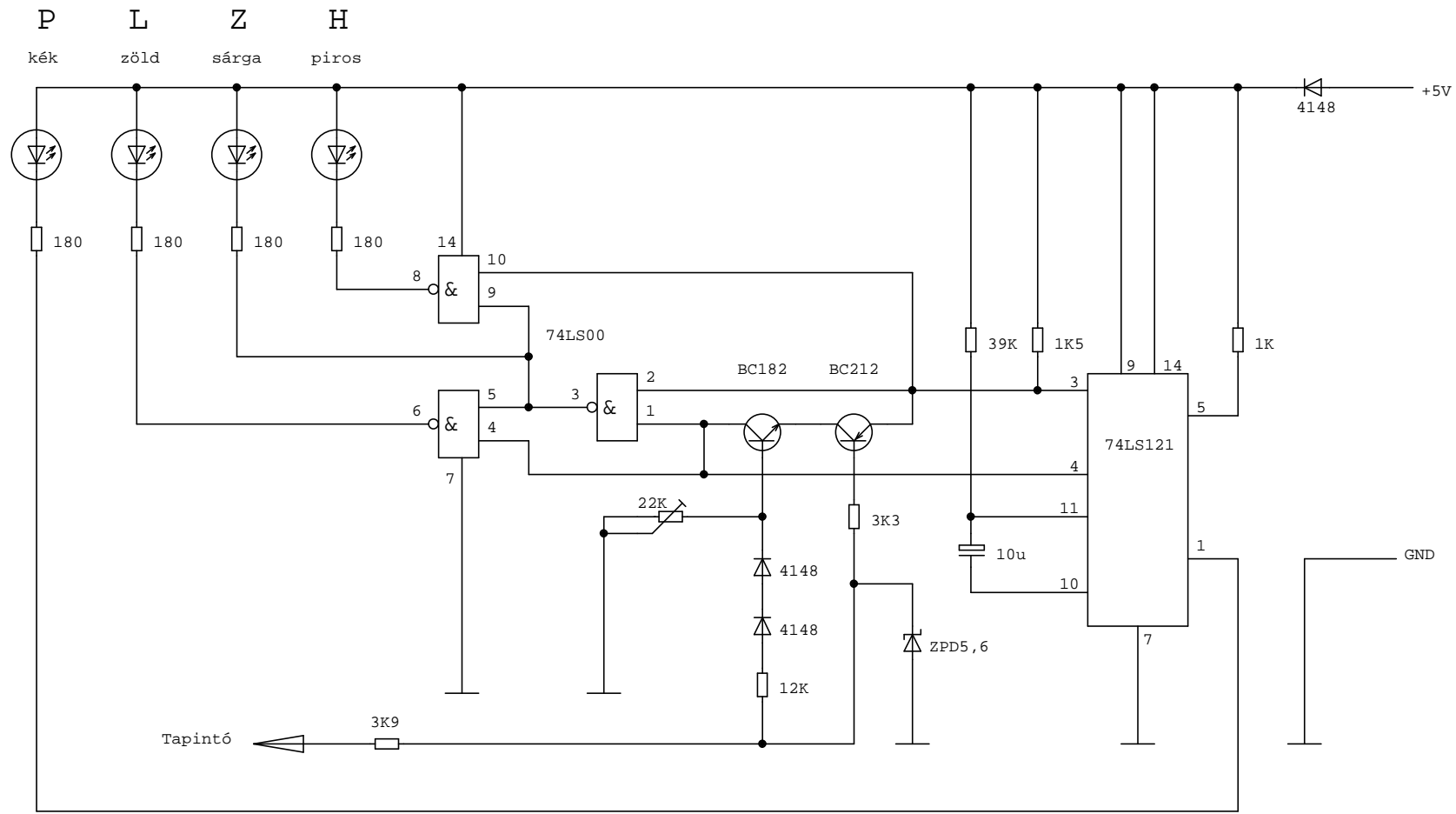
Logikai teszter Csak TTL !!
