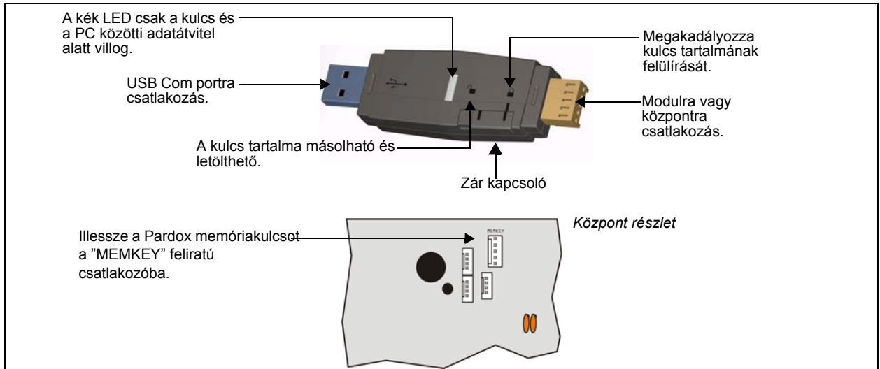
7. ábra: Paradox Memóriakulcs
