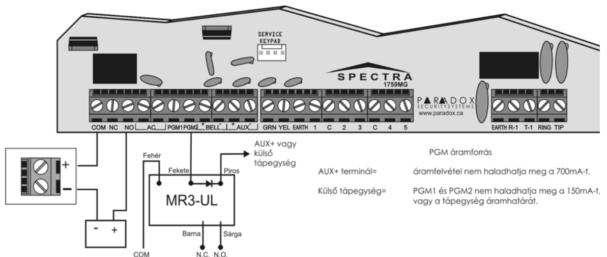
2. ábra: Relé és PGM bekötések
