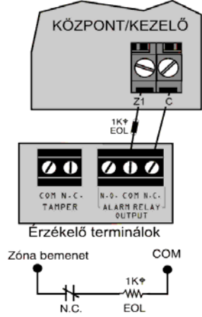
3. ábra: Szimpla zóna bemenet bekötések
