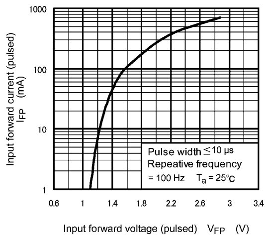
Fig. 11.6 I_{FP} - V_{FP}
