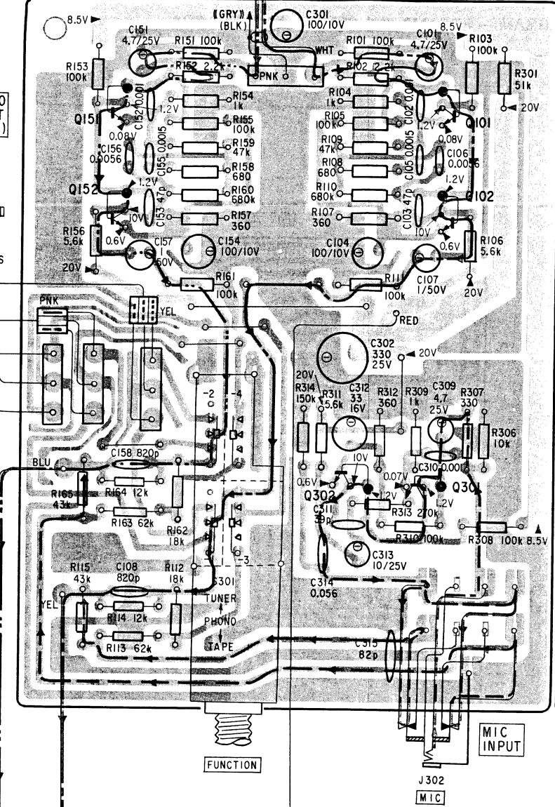
【PREAMP BOARD】 (COMPONENT SIDE)
