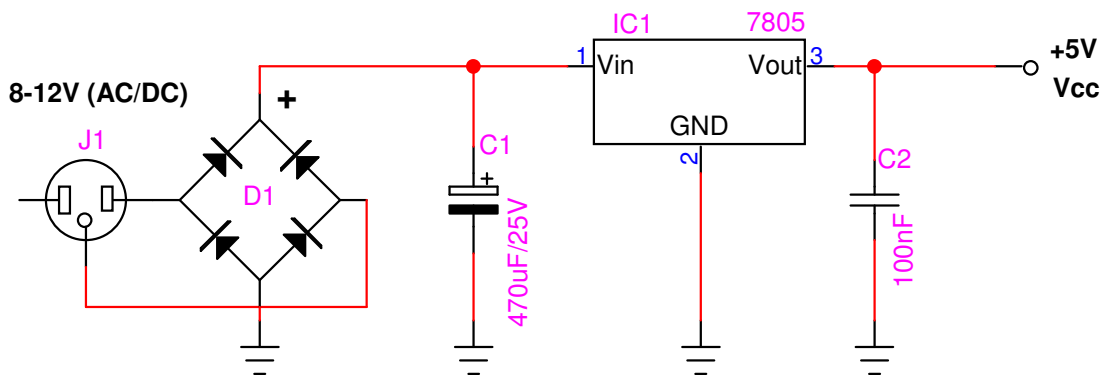
1. ábra 5V-os tápegység
