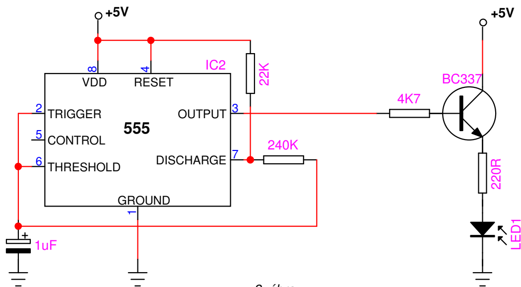
2. ábra Oscillátor
