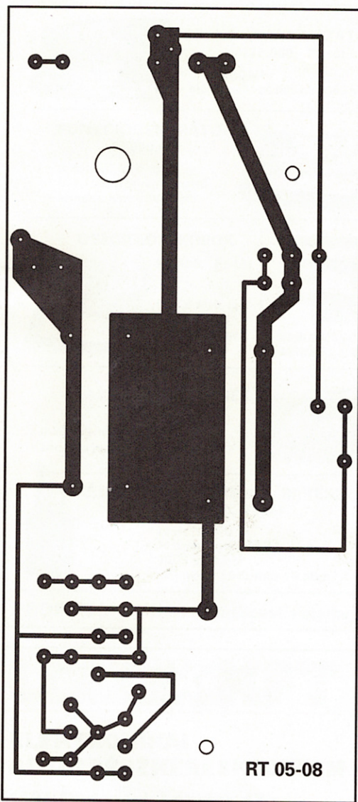
Tápegység a híderősítőhöz
