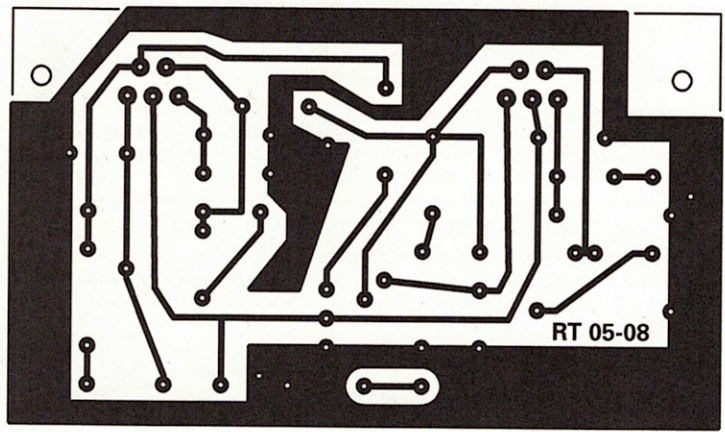
Híderősítő
