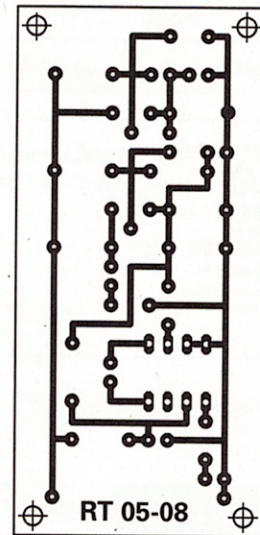
Pixie-2 adó-vevő
