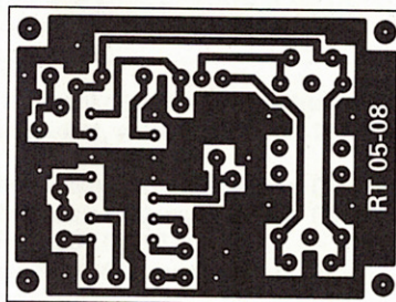
DRM-konverter
