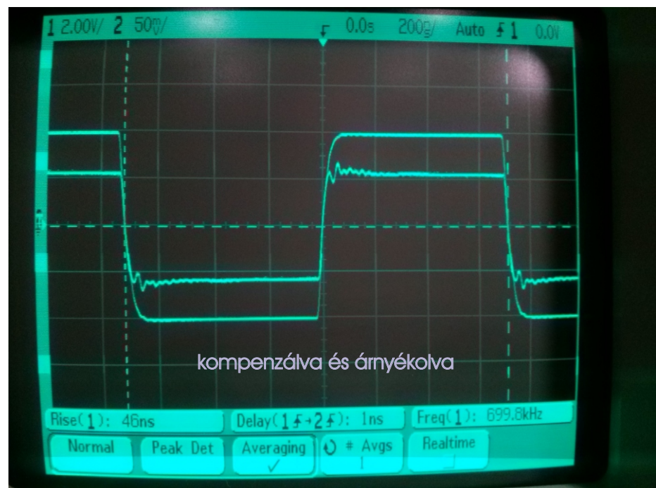
Reed-relés feszültségosztó négyzetjel átvitele (-37 dB) f=700 kHz
