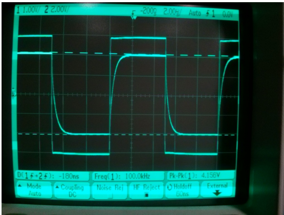
U_{be} = 12 \text{ Vpp} U_{ki} = 4.15 \text{ Vpp} relék fesz. osztása = -21 dB
