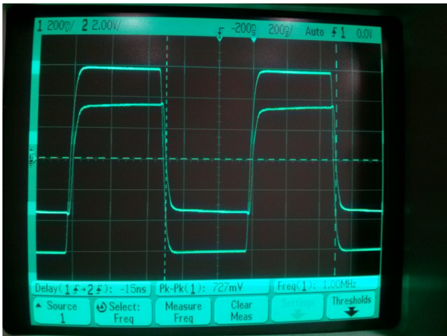
U_{be} = 12 \text{ Vpp} U_{ki} = 727 \text{ mVpp} relék fesz. osztása = -37 dB
